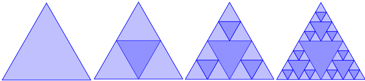
Figura 1 - Triângulo de Sierpinski
