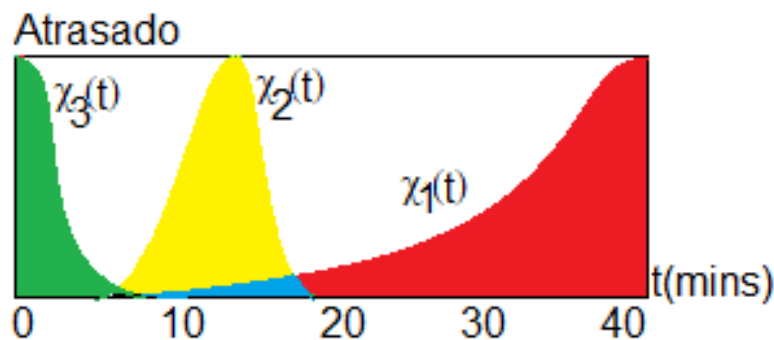
Figura 5 A operação de “e lógico” entre as funções de pertinência “medianamente atrasado” e “muito atrasado” representada pela área azul
