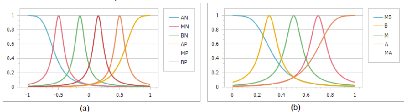
Figura 6 As funções de pertinência para as variáveis difusas do problema. A Figura 6a se refere às funções de pertinência de ME e IA, enquanto a Figura 6b se refere às funções de pertinência das variáveis difusas CN e CP
