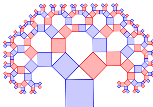
Figura 7 Árvore Pitagórica Isósceles Regular
